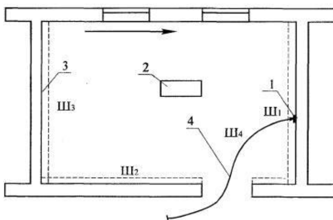
Рис. 26. Схема организации рабочего места звена № 1
